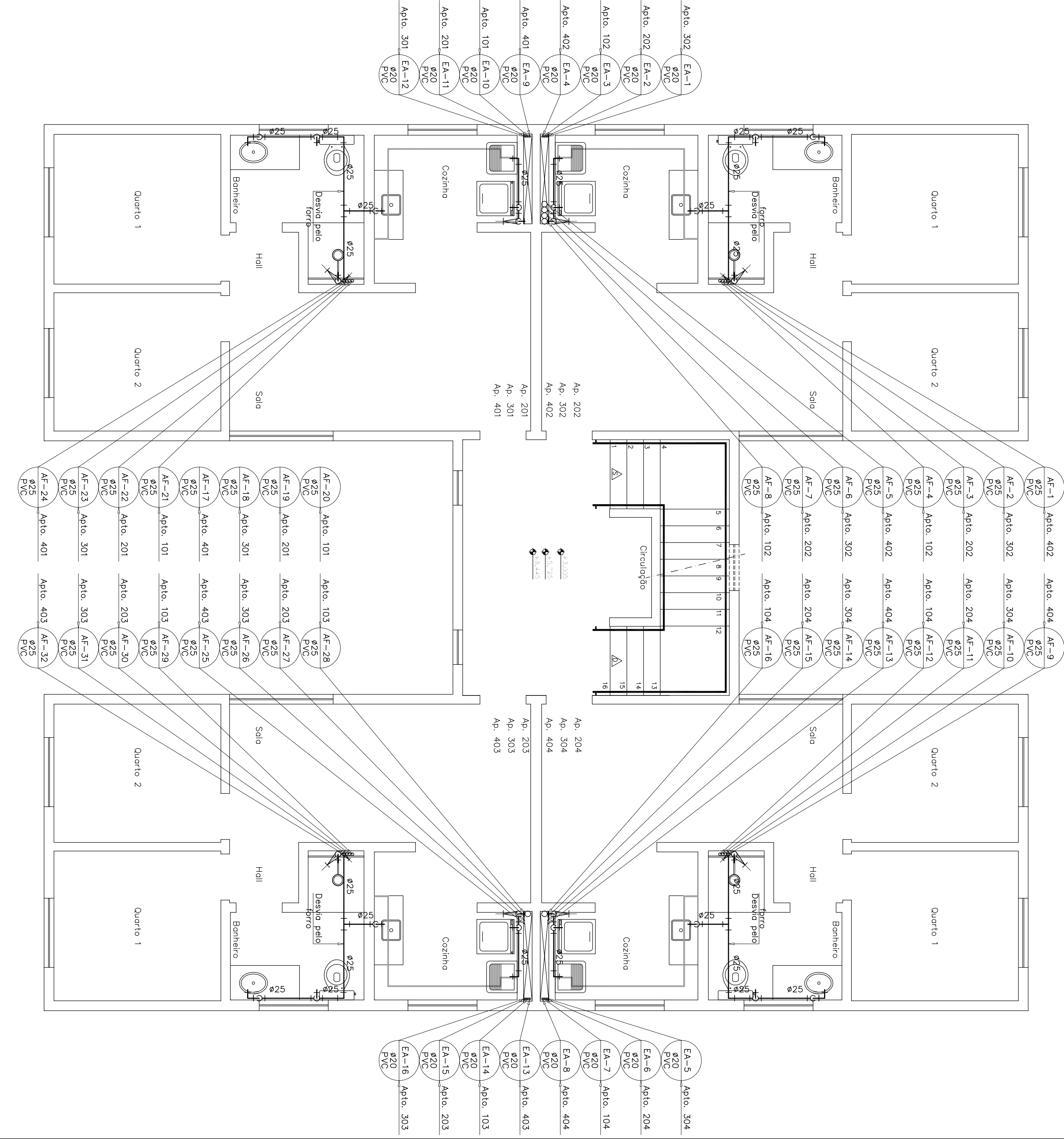
PLANTA DO PAVIMENTO TIPO – ÁGUA POTÁVEL
