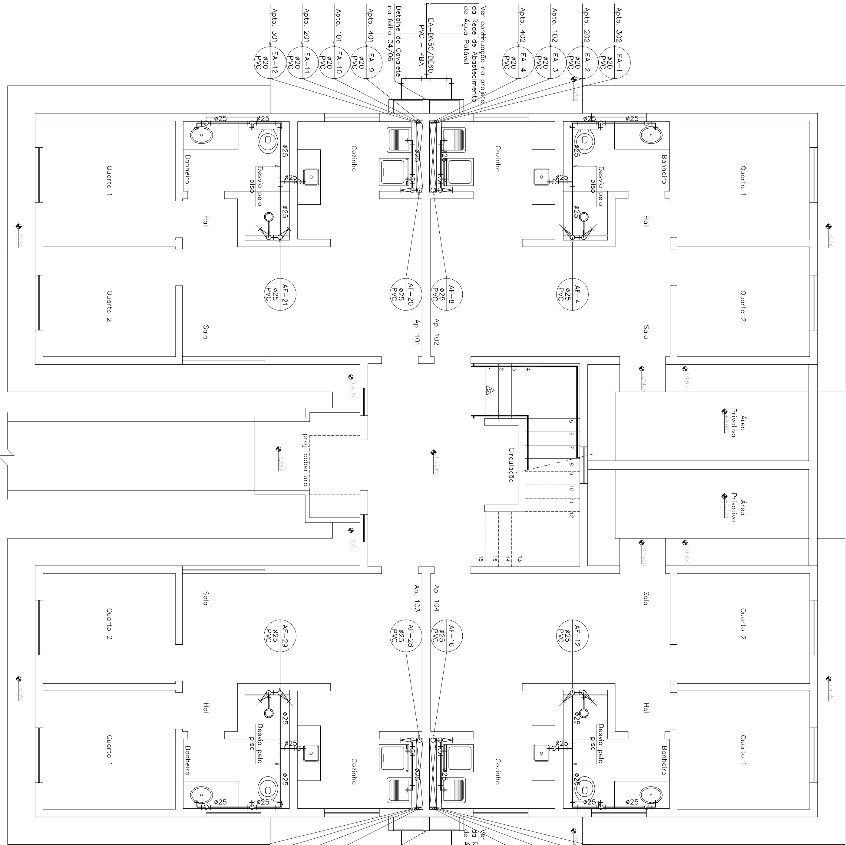
PLANTA DO PAVIMENTO TERREO – ÁGUA POTÁVEL
